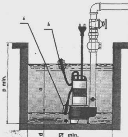
Типовая установка однофазного насоса
